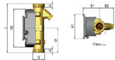
Abmessungen qp 1.5 - 2.5
