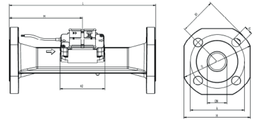
Abmessungen qp 15.0
