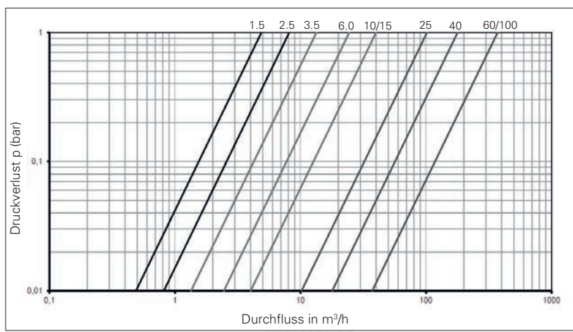
Druckverlustkurve
