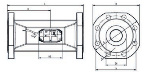
Abmessungen qp 25.0 - 100.0
