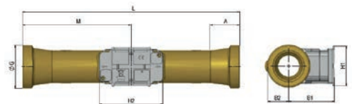
Abmessungen qp 3.5 - 10.0
