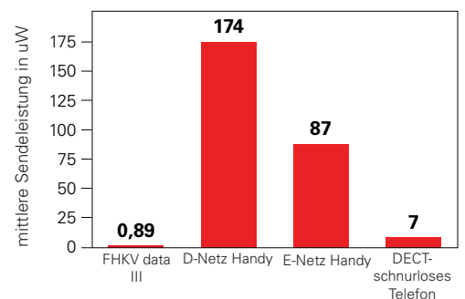
Mittlere Sendeleistung unterschiedlicher Funksender im Vergleich mit dem Funk-Heizkostenverteiler data III
