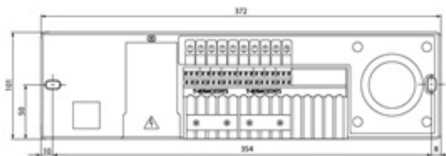
Hauptregler Danfoss Icon™ 24V
