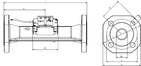
Abmessungen qp 15.0
