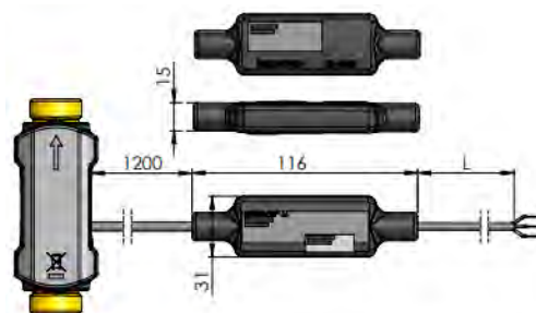
Elektronikbox
