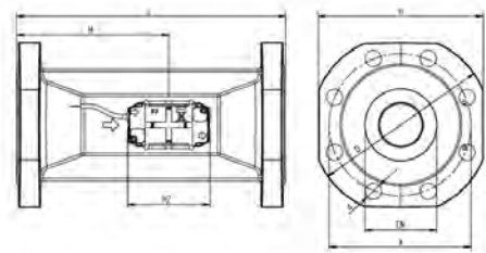
Abmessungen qp 25.0 - 100.0
