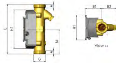
Abmessungen qp 1.5 - 2.5
